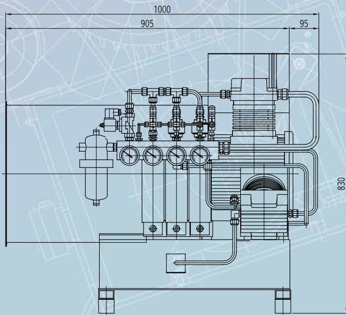
Vista laterale del tipo WTEG, versione tristadio
